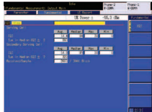
CQI
