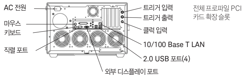
그림 9. 16800시리즈 후면판
